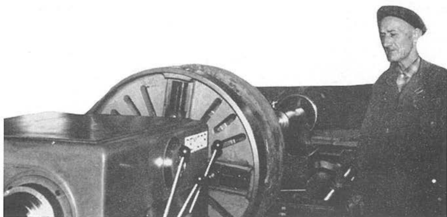
Verkstedet har fått ny dreiebenk, dreielengden er 6 meter. Prisen var kr. 100.000 , den er av fabrikat Demoor ( Belgisk ). Sigurd Nordal betjener dreiebenken.
